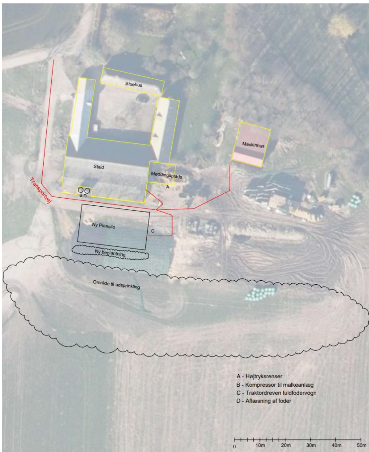
Figur 3: Situationsplan, der viser bygninger, anlæg og udsprinklingsområde på ejendommen. Jævnfør ansøgningsmateriale.
