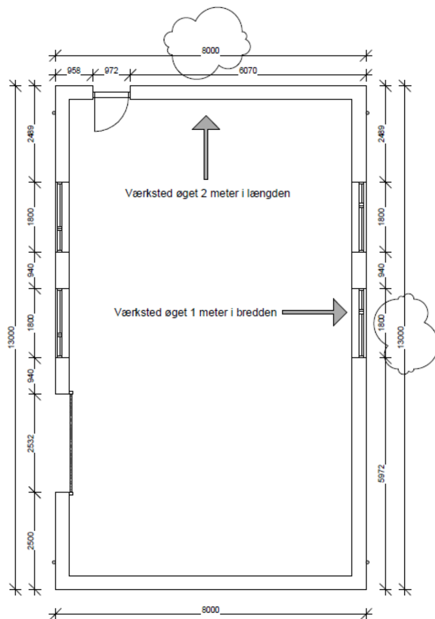
Ansøgers indsendte plantegning af det ansøgte projekt
