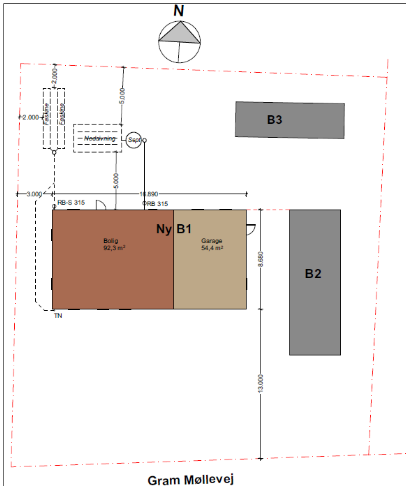
Ansøgers indsendte situationsplan
