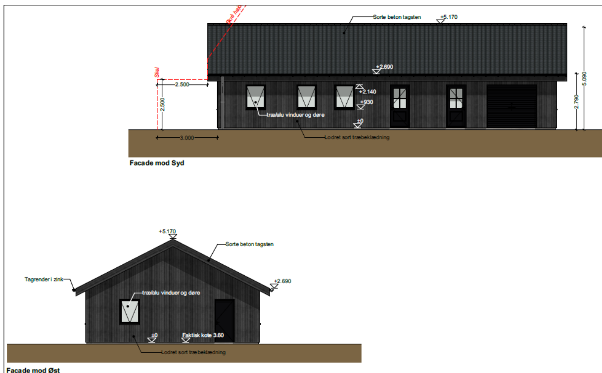
Ansøgers indsendte facadetegetninger
