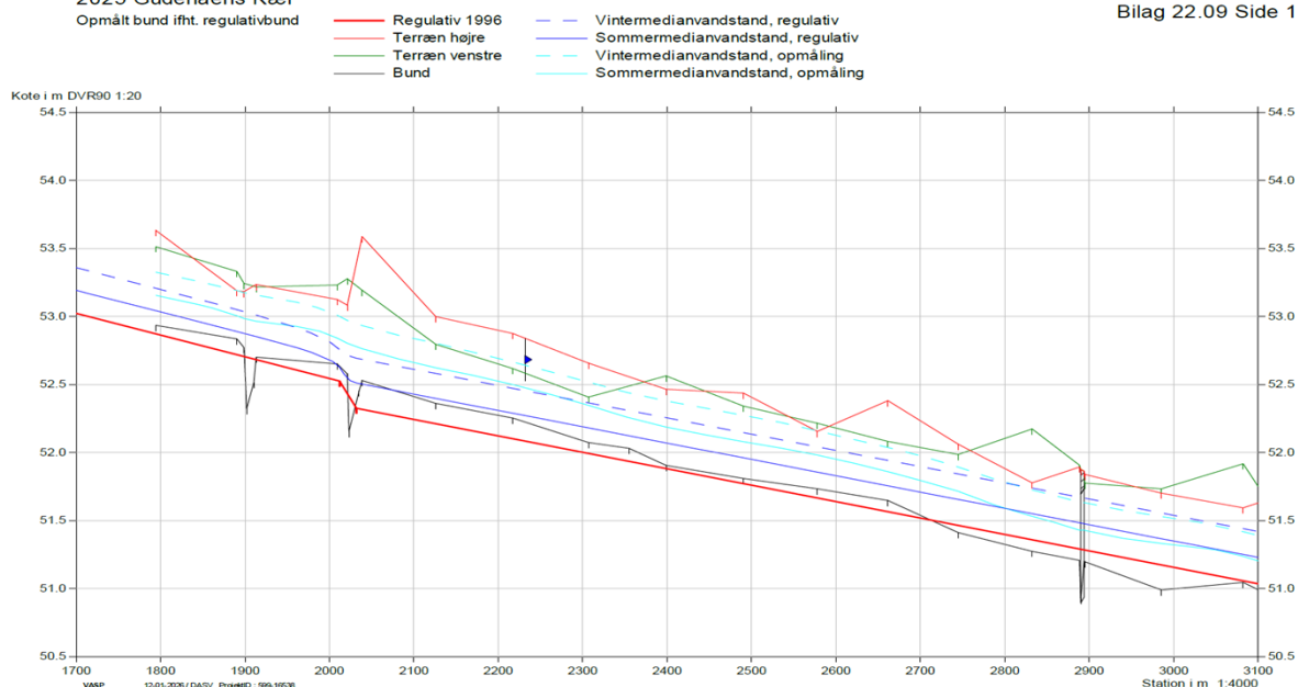
Figur 2. Opmåling af bund i Hjortsvang-Tørring Bæk
