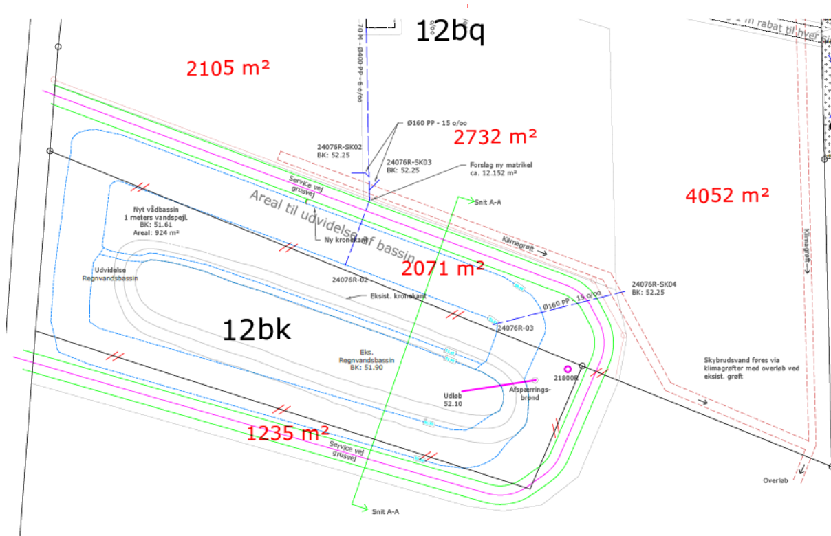
Figur 2. Tegning af bassinudformning fra ansøgningsmaterialet.
