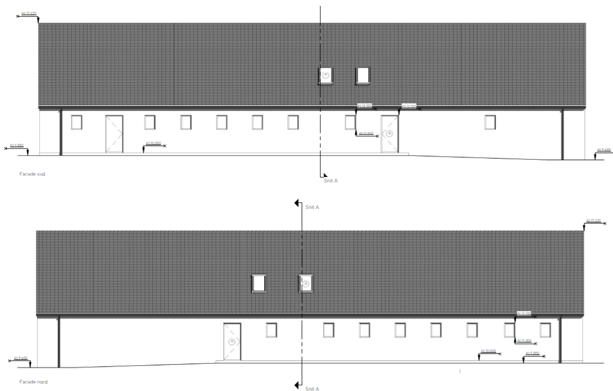
Ansøgers indsendte tegninger af facaderne mod syd og nord
