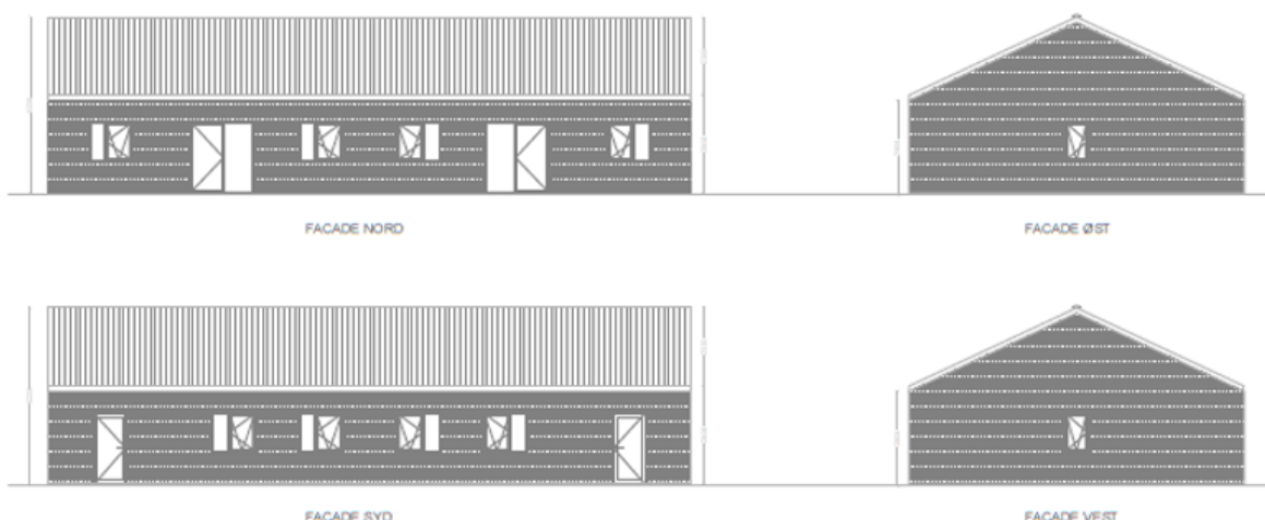
Ansøgers indsendte facadetegninger af det ansøgte projekt
