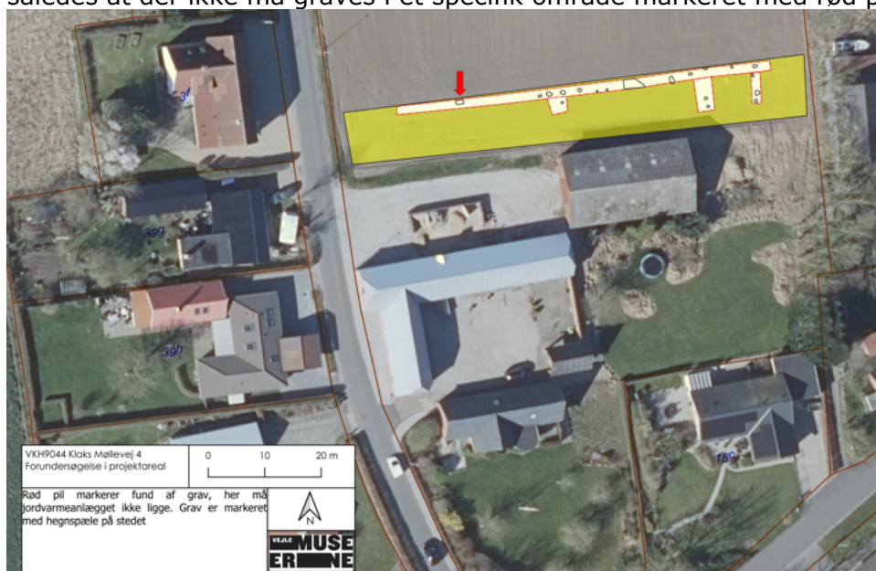
Figur 1 Område, hvor nedgravning af jordslanger ikke er tilladt, er markeret med rød pil
