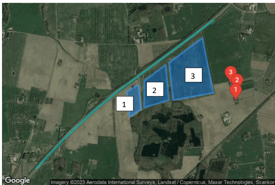
Figur 4 Forenklet modellering i Forge Solar værktøjet. Nærmeste vej (E45) og observationspunkter er markeret.
