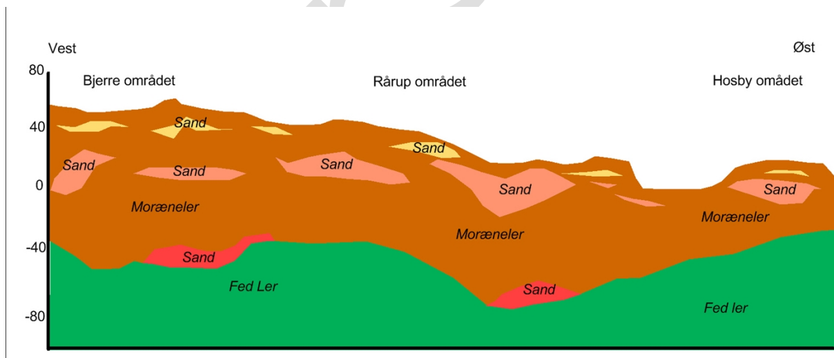
Figur 8.5. Principskitse for de geologiske forhold
