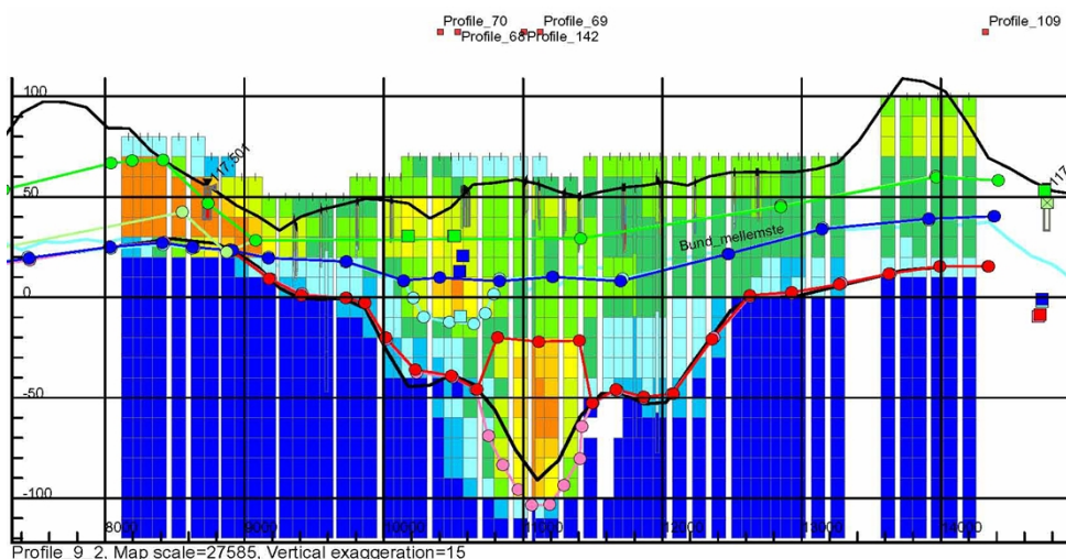
Figur 8.4. Eksempel på profilsnit fra den geologiske model
