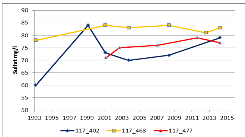
Figur 6: Udviklingen i nitrat- og sulfatindholdet i boringerne.
